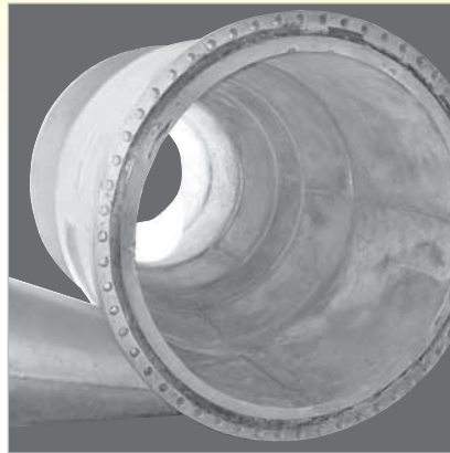
KALSICA-N Zyklon mit 1 200 mm Durchmesser für Siliziumsand
