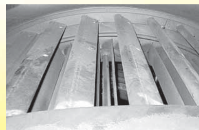
Leitschaufeln des Sichters einer Kohlemühle aus KALSICA-A
