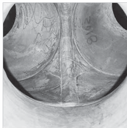
Mit KALSICA Formteilen ausgekleidete Rohrweiche
