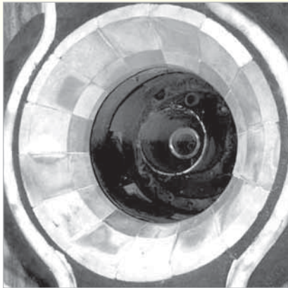
Brenner-Konus im Kraftwerk aus KALSICA-N
