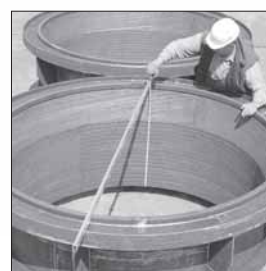
Abscheidekonen von Zementsichtern aus KALMETALL-W 100 6+4, Durchmesser 3 000 mm
